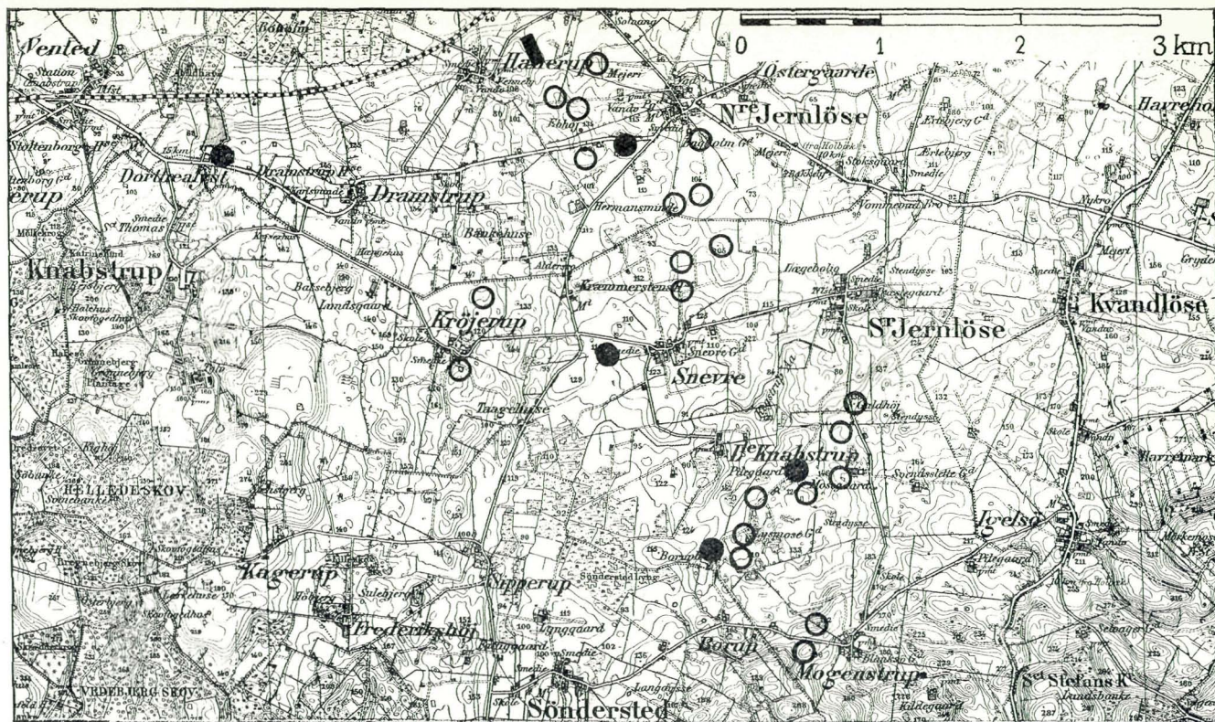
Fig. 1. Kort over Forekomsten af paleocæn Mergel i Hanerup Omraadet. Den sorte Rektangel Nordøst for Hanerup angiver Beliggenheden af den store Grav. Cirklerne de øvrige Forekomster (se S. 394). Højdekurverne er 10 Fods Kurver. Maalestoksforholdet ca. 1:48500. Efter Generalstabens Atlasblade Tølløse og Jyderup.
