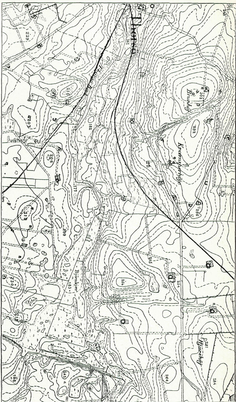
Fig. 2. Spalddale mellem Thorsø og Havrum.
