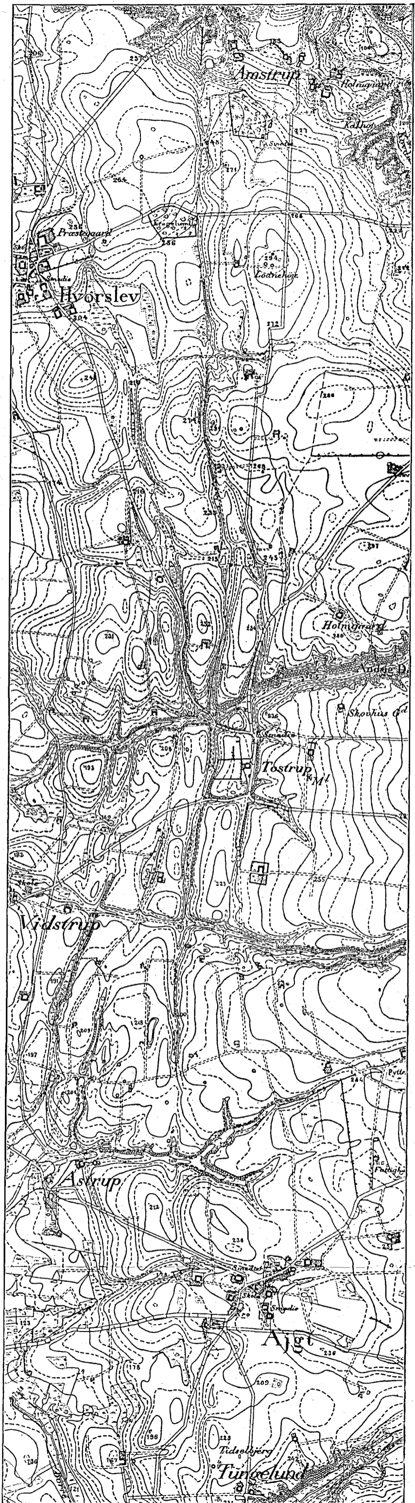
Kort over Spaltedale mellem Amstrup og Tungebund.
