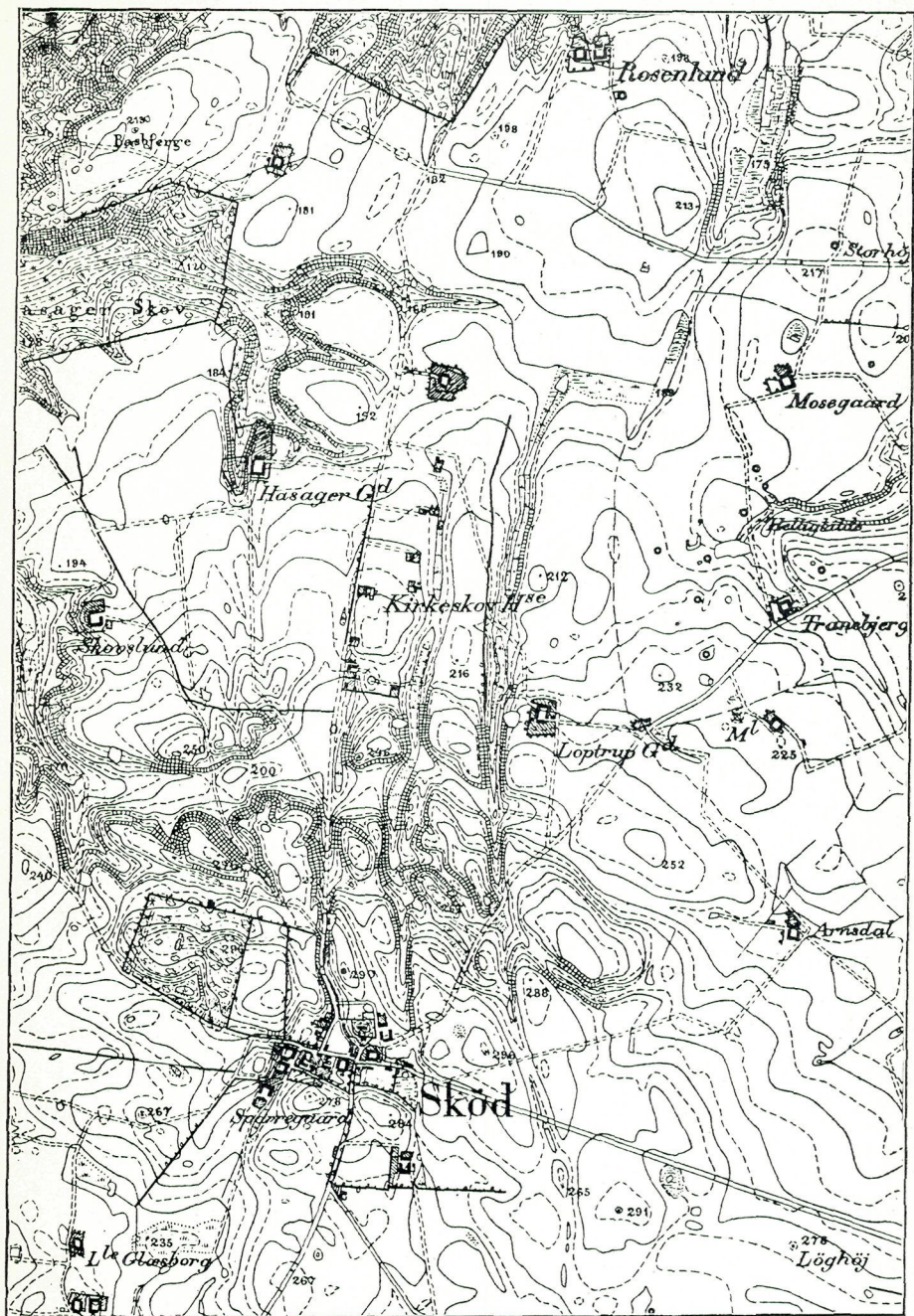
Fig. 3. Spaltdale omkring Sköd.
