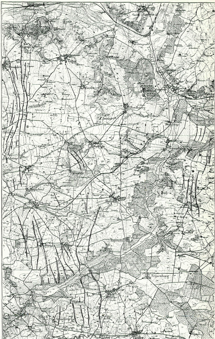
Fig. 1. Kort over Spaltedalenes Beliggenhed. Maalestok 1 : 100,000.
