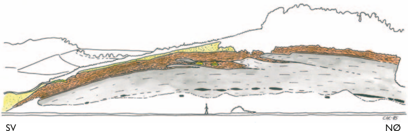
Fig. 20. Silstrup Sydklint. A , Fur Formationen overlejres af brunt oligocænt ler (Sydklint Led, Brejning Formationen) med et tyndt grønt, glaukonitisk bundlag. Midt i klinten ses glacialtektoniske overskydninger, mens der andre steder i klinten er uforstyrret sedimentær kontakt mellem Eocæn (grå) og Oligocæn (brun), se Fig. 21. B , Kun blottede lag er farvelagt (det gule er kvartært sediment). De sorte linser i klinten er cementstenen ved +135. På stranden ses en person som skala. Foto og tegning Claus Heilmann-Clausen.
