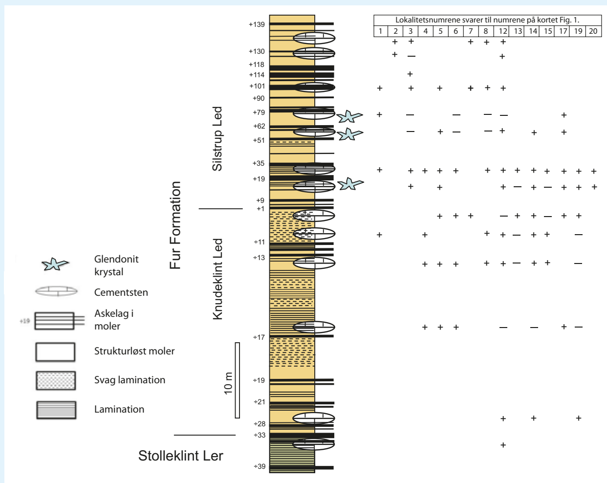
Fig. 33. Forekomsten af cementsten og glendonitkrystaller i Fur Formationen. Simplificeret log med angivelse af cementstens-niveauer i Fur Formationen. Bemærk at glendonitkrystallerne findes mellem askelag +3 og +79, og at krystallerne kun i nogle tilfælde er indesluttet i cementsten. Bemærk at der er fem niveauer, som altid har cementsten (se teksten), og at de øvrige niveauer kun optræder på én eller få lokaliteter.
