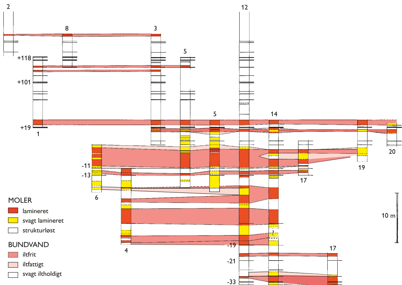
Fig. 27. Vekslen mellem perioder med iltfrit, iltfattigt og svagt iltholdigt bundvand. Læg mærke til, at skiftene er stort set samtidige gennem hele bassinet. De vigtigste askelag er angivet (fra –33 til +118). Tallene ved lagsøjlerne refererer til lokaliteternes numre på Fig. 1 (efter Pedersen 1978, 1981).
