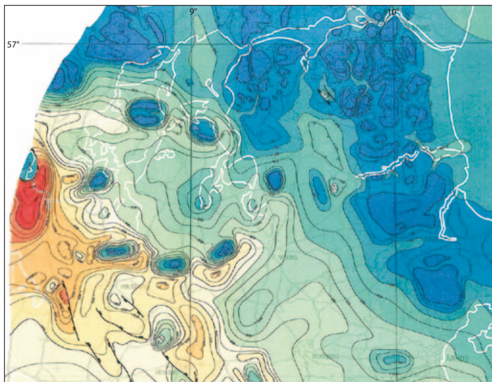
Fig. 3. Kort over dybden til kalkoverfladen i Nordjylland. Kurvækvidstanden er 25 m mellem +50 og -50 m, herunder 50 m ækvidistance. Bemærk at kalkoverfladen ligger højt over salt diapirerne (blå farve) og dybt mod syd og vest (gullige farver). Tykt optrukne, sorte streger er normalforkastninger, de sorte rektangler viser den nedforkastede blok. Efter Ter-Borch 1991.
