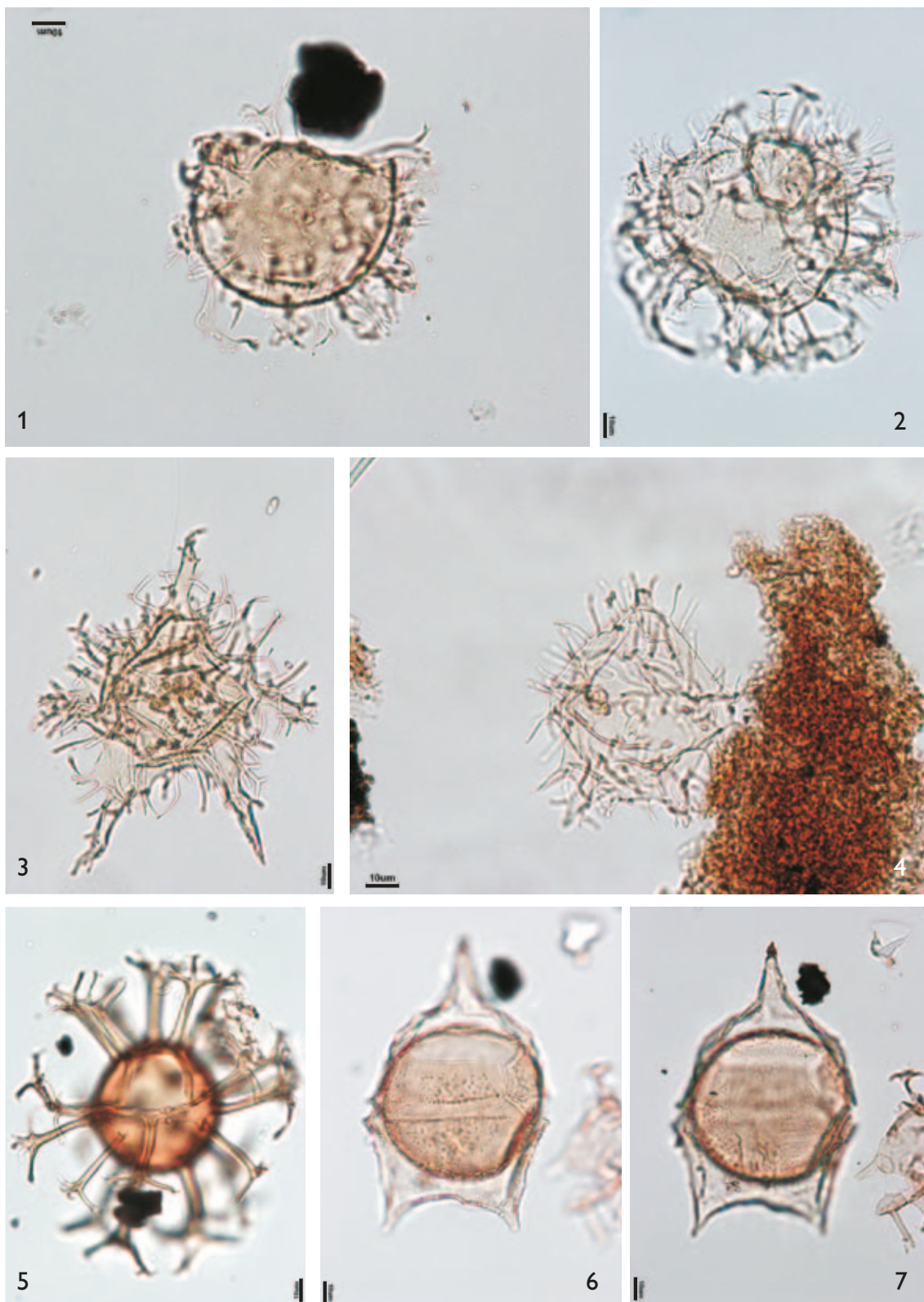
Fig. 49. Organisk-væggede dinoflagellatcyster fotograferet i normalt lysmikroskop, skala = 10µm. For alle arter er der givet følgende oplysninger: a) Artsnavn, b) Lokalitet (St= Stolleklint, Sy= Silstrup Sydklint) og prøvenummer. Prøverne stratigrafiske indplacering findes i Willumsen (1997; 2004: Fig. 3). 1, Glaphyrocysta ordinata , St25; 2, Glaphyrocysta cf. divaricata , St51; 3, Apectodinium cf. parvum , St12; 4, Apectodinium quinquelatum , St12; 5, Achomospaera alaicornu , Sy10; 6 og 7, Deflandrea oebisfeldensis , Sy10. Foto Pi Suhr Willumsen.
