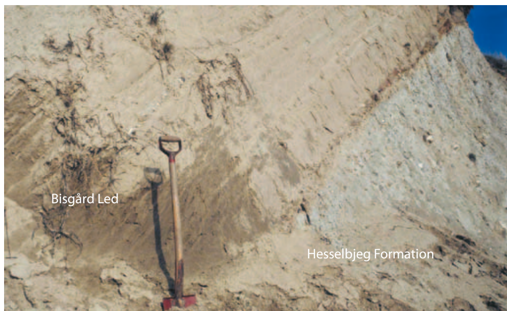
Fig. 56. Hesselbjerg formationen overlejres af glaciolacustrint ler og finsand tilhørende Bisgård led, Vilsund formationen. På grund af glacialtektonisk deformation hælder lagserien mod nord (venstre i billedet). Kystklint på Mors, ca. 1,6 km syd for Vilsundbroen. Foto Stig Schack Pedersen.
