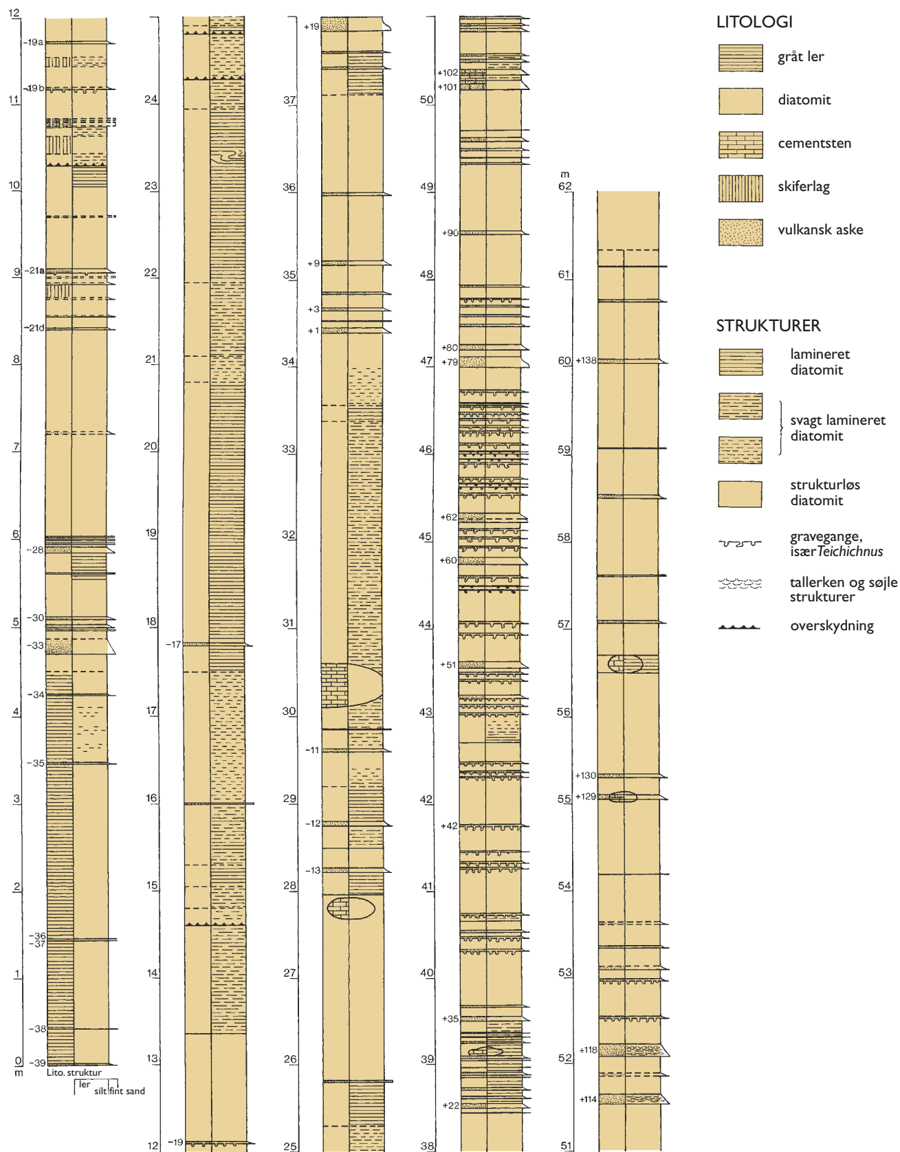
Fig. 18. Sedimentologisk log gennem Fur Formationen (Pedersen & Surlyk 1983). De nederste 4,5 m blev betegnet de molerliggende overgangslag ved opstillingen af Fur Formationen (Pedersen & Surlyk 1983), og henføres nu til Stolleklint Leret.
