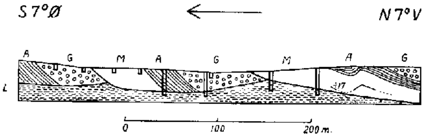
Fig. 4. Tværprofil af Molerområdet ved Sundby. L: sort Ler og leret Moler, M: negative Molerserie, A: positive Molerserie (Askeserie), G: Diluvialgrus.
