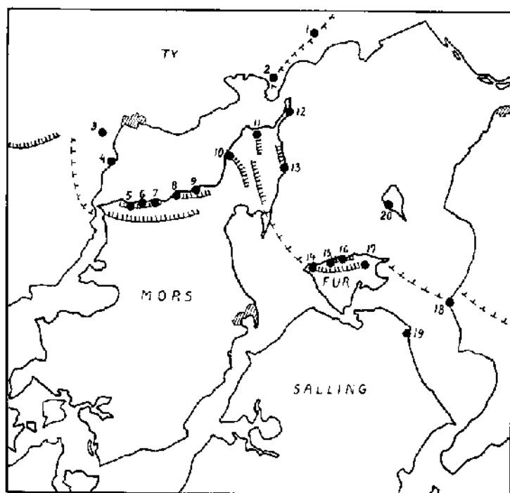
Fig. 2. Kort over Egnen omkring Mors (1:500000). Randmoræner og formodede Randmoræner væsentlig efter N. V. Ussing; Molerforekomster efter O. B. Roggild. 1. Vesløs, 2. S. Arup, 3. Titsted, 4. Silstrup, 5. Sundby, 6. Svalklit, 7. Gullerup, 8. Hanklit, 9. Salgjerhøj, 10. Skærbæk, 11. Skarreluge, 12. Feggeklit, 13. Ejerslev, 14. Knuden, 15. Stollcklint, 16. Fur Østklint, 17. Færker, 18. Ertbølle, 19. Junget, 20. Livø.
