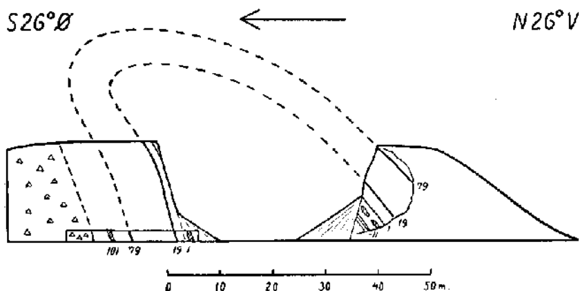
Fig. 5. Tværprofil af Gullerup Molerbrud.
