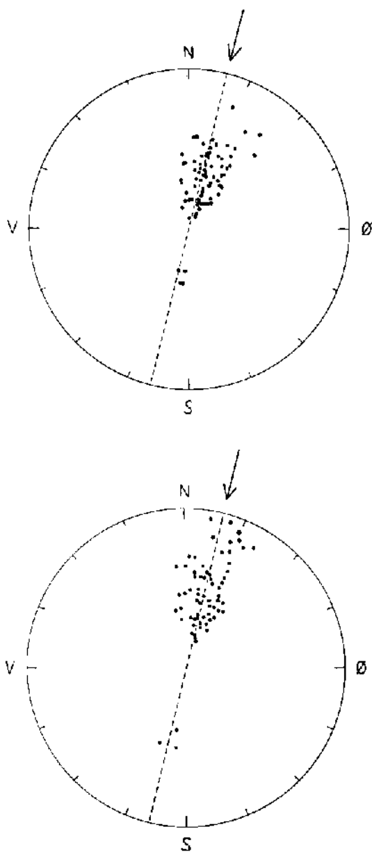
Fig. 20. Stereografisk Projektion af Lagstillingerne (føroven) og Overskydningsfladerne (førueden) i Løstrup Klint (Axel Jessens Opmaalinge). Zonekredsen stiplet. Pilen markerer Istrykkets Retning.
