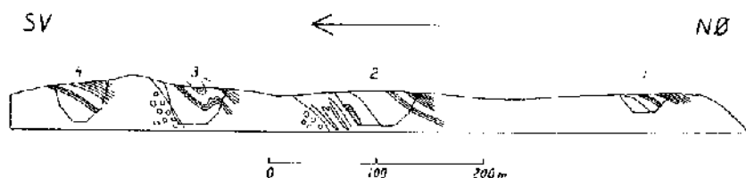
Fig. 16. Skitse af Snit gennem Knuden, Fur, med de 4 Molergrave. Streget: positive Molerserie, derunder 3 Streger: —11— 13. 1 Streg: —17. Folderne til venstre i Grav 2 er —33. Ringe markerer Diluvialgrus. Se ogsaa Fig. 17 og 17a.
