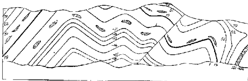
Fig. 9. Klinten ved Skærbæk (O. B. BOGGILD) Istryk fra venstre.
