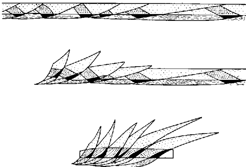
Fig. 21. Principet for Dannelsen af Lønstrup Klint og andre dislocerede Klinter af lignende Art. Istryk fra venstre. Øverste Figur viser den Stilling, Flagerne mellem Pæl 43 og 45 maa antages at have indtaget inden Forstyrrelserne. Prikket: Diluvial sand (de i Klinten nu synlige Dele kraftigt prikket), streget: Diluvialer (det i Klinten synlige: sort) Midterste Figur: Sammenskydningen er begyndt nærmest Isen. Nederste Figur: Flagernes nuværende Stilling.
