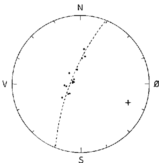
Fig. 1. Stereografisk Projektion af Maalinger af Lagstillinger ved Ertbølle. Indtegnet Zonekreds (----) og Zoneakse (Foldningsakse) (+).
