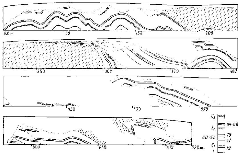
Fig. 13. Tværprofil af Feggeklit (Skitse). Streget Areal: Morænedannelser, overvejende Moræneler; hvidt Areal: bevokset; C_1 - C_3 som i Fig. 5. Istryk fra venstre.
