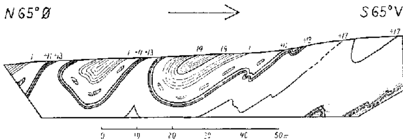
Fig. 11. Tværprofil af Skarrehage Molergrav. Den lille Skiferfold svarer til den venstre Fold i Fig. 10, Skiferlagene til højre til en Del af højre Fold.
