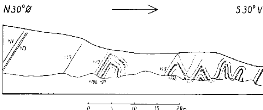
Fig. 19. Skitse af Profilet med Knudefolderne. Skraverede Daand markerer Skiferlag.
