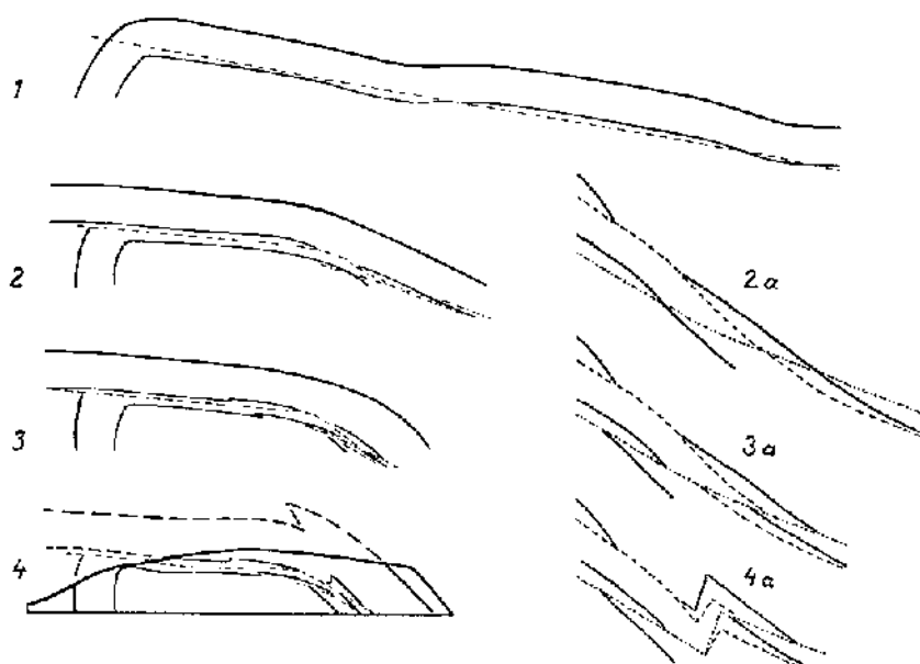
Fig. 8. Udviklingen af Forstyrrelserne i Firkanten ved Silstrup. Af de to fuldt optrukne Linjer betegner den nedre Lagene omkring 60—62, den øvre Cementstenen med 101 og 102. --- er den store Overskydningsflade, ---- Underskydningsfladen. Fig. 2a—4a viser i større Maalestok Princippet for Forstyrrelserne i den østlige Del af Klinten (mellem 90 og 105 m i Fig. 7). I Fig. 4 er indtegnet den nuværende Klintoverflade og alt over denne er stipleet.
